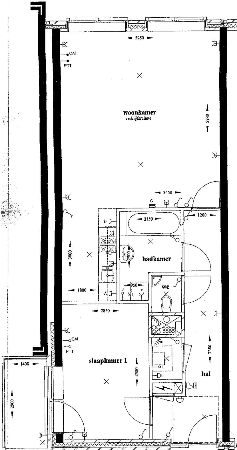
APPARTEMENT 1E VERDIEPING, NR. 1 © APPARTEMENT 2E VERDIEPING, NR. 6 APPARTEMENT 3E VERDIEPING, NR. 11
